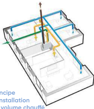
Principe d'installation en combles
